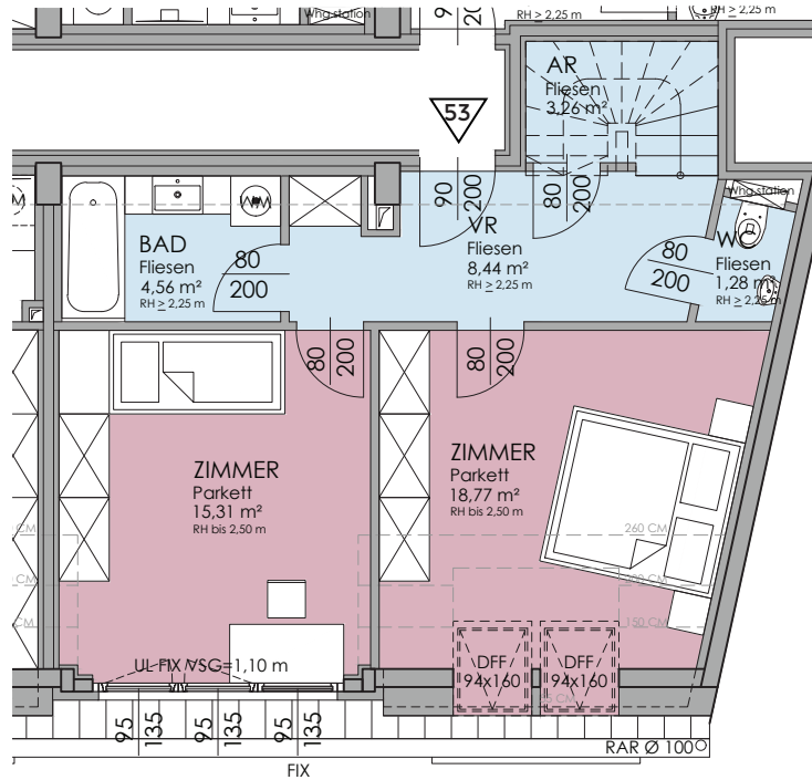
1. Dachgeschoß
