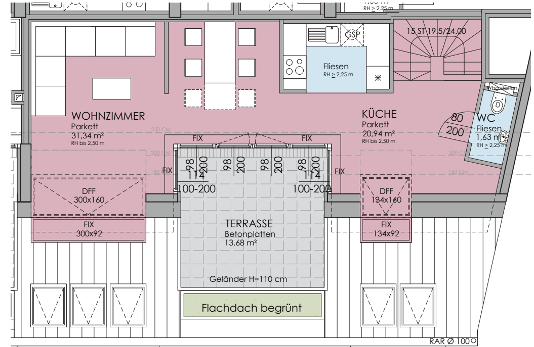
TOP 53 1.+2. Dachgeschoß
