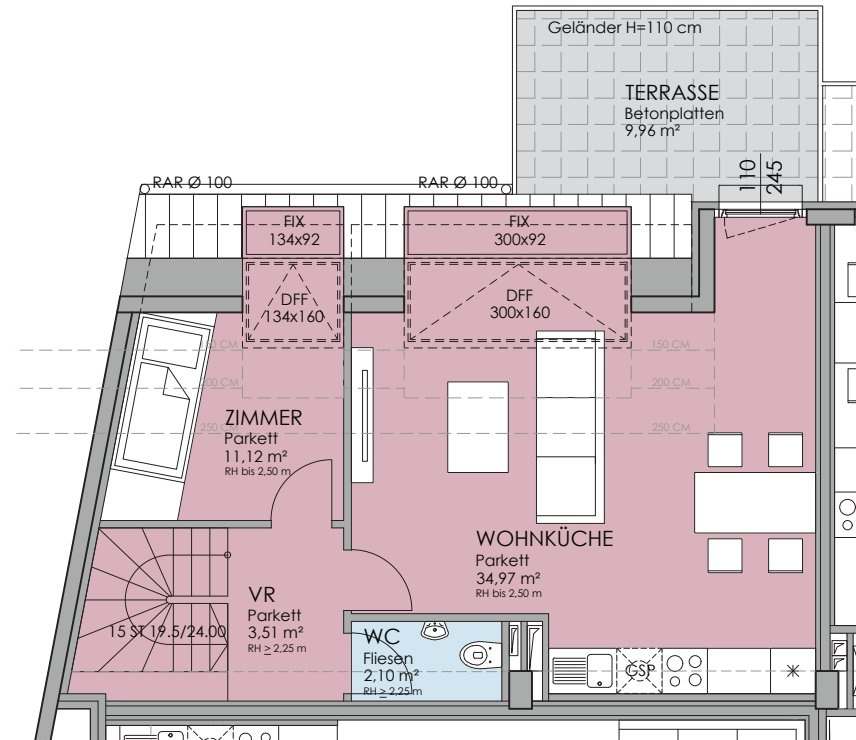
TOP 59 1.+2. Dachgeschoß
